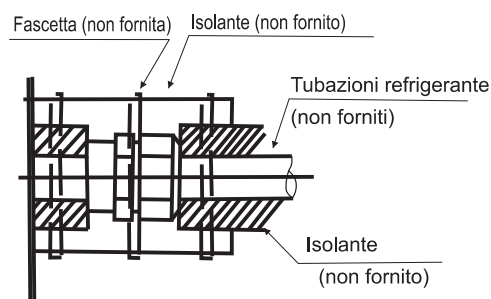
Procedura di isolamento delle tubazioni
