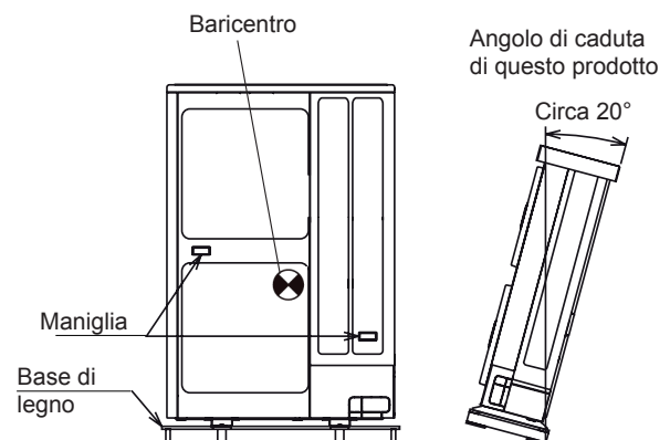
Fig. 3.2 Movimentazione dell'unità esterna
