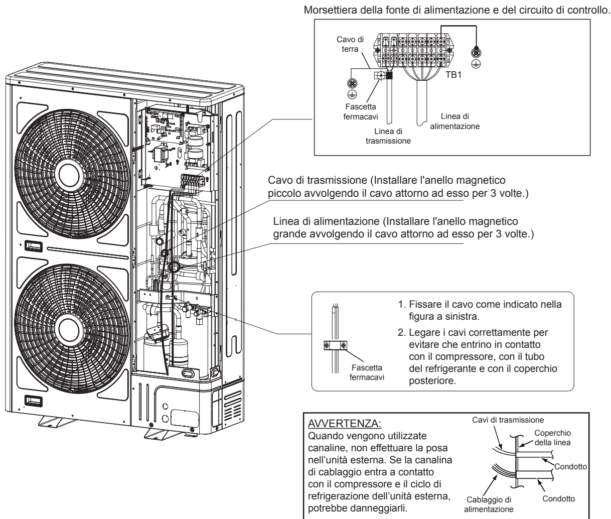
Fig. 6.2 Collegamenti elettrici dell'unità esterna
