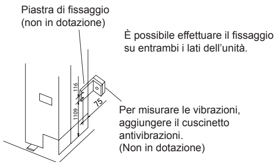
Fig. 4.3 Ulteriori indicazioni per il fissaggio
