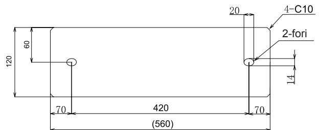
Fig. 4.4 Installazione di telaio e base
