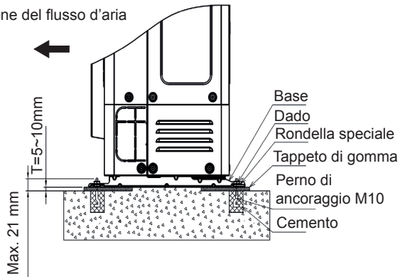
Fig. 4.1 Installazione dei perni di ancoraggio
