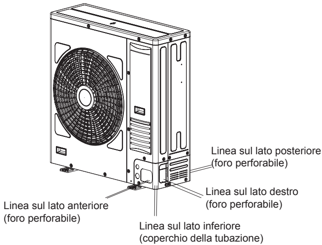
Fig. 5.1 Direzione delle tubazioni
