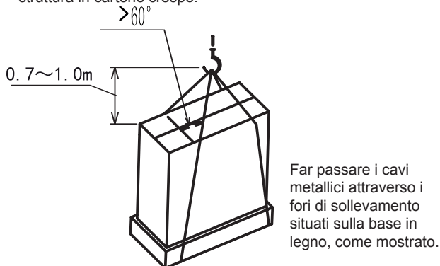
Fig. 3.1 Operazioni di sollevamento per il trasporto
