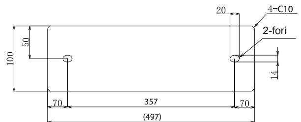
Fig. 4.6 Installazione di telaio e base
