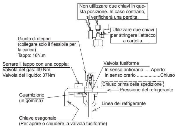
Coppia della valvola fusiforme (Nm)
