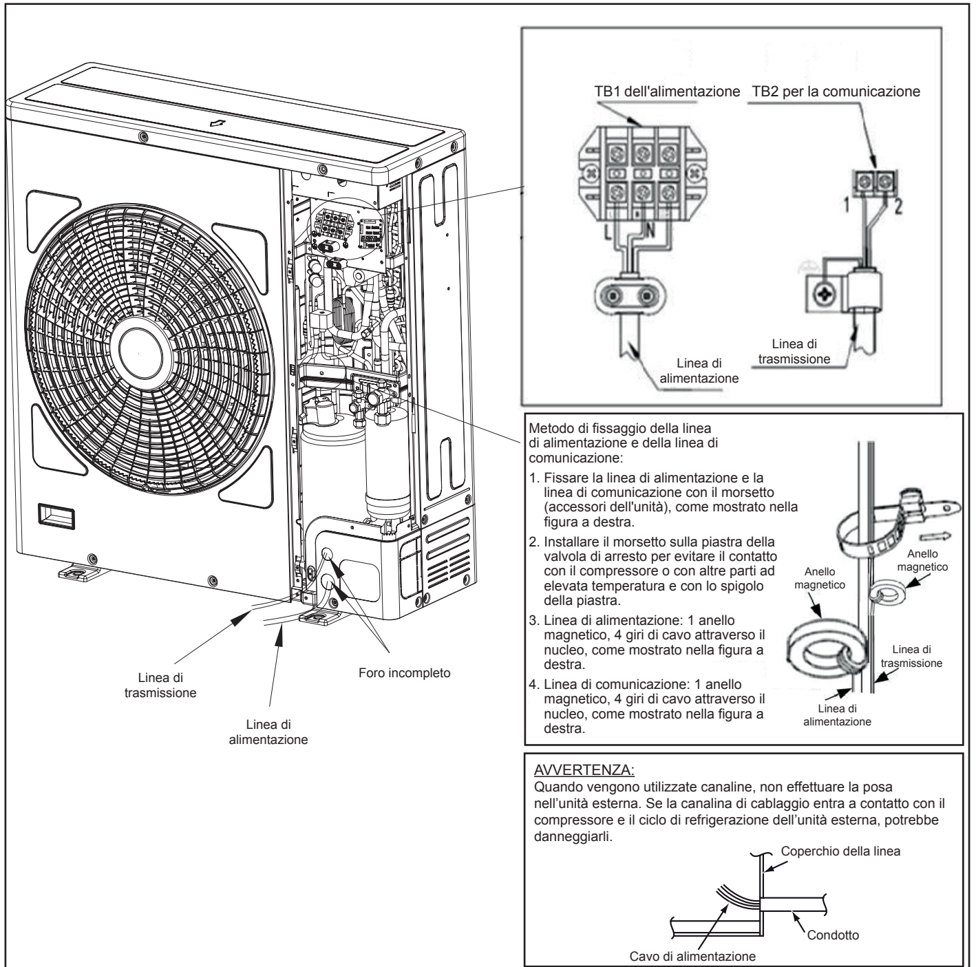
Fig. 6.3 Collegamenti elettrici dell'unità esterna
