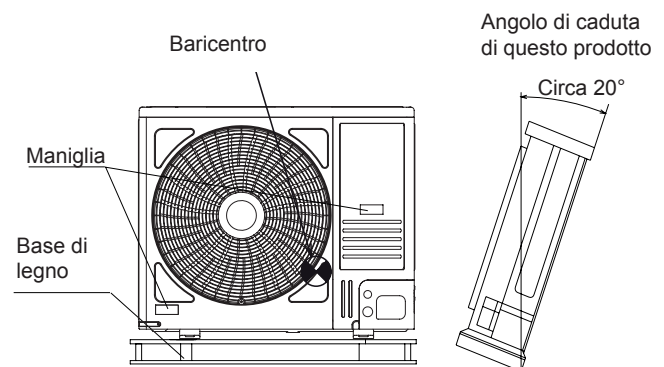
Fig. 3.2 Movimentazione dell'unità esterna
