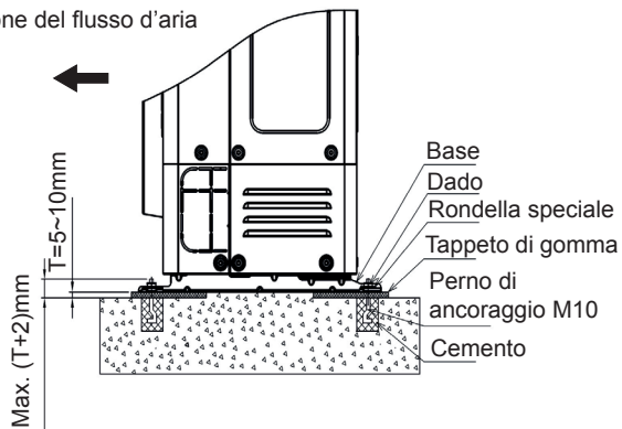
Fig. 4.2 Installazione dei perni di ancoraggio
