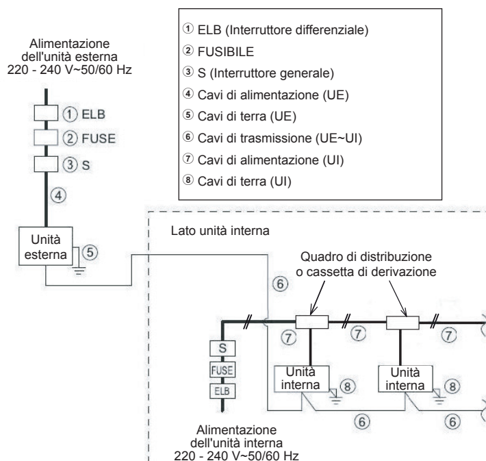
Fig. 6.2 (a) Collegamenti elettrici (220 - 240 V ~ 50/60 Hz)
