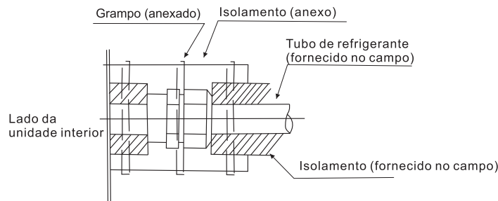
Fig. 4.4 Procedimento de isolamento da tubagem
