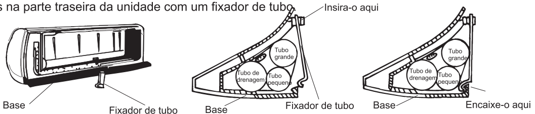
A. Insira o fixador de tubo para a ranhura. B. Pressione para ligar o fixador de tubo para a base. C. Encaixe o tubo de drenagem na ranhura.
