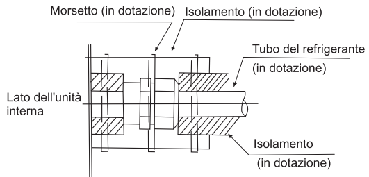
Fig. 4.5 Procedura di isolamento dei tubi
